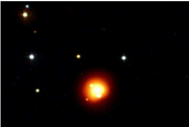
GRB 080916C 16-sept-2008 ( + 12.2 milliards a.l.) La plus violente explosion jamais encore observée. 5 masses solaires transformées en X et γ en 60 secondes
